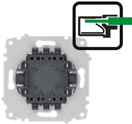
Quick Connect (screwless) Hızlı Bağlantı (vidasız)
